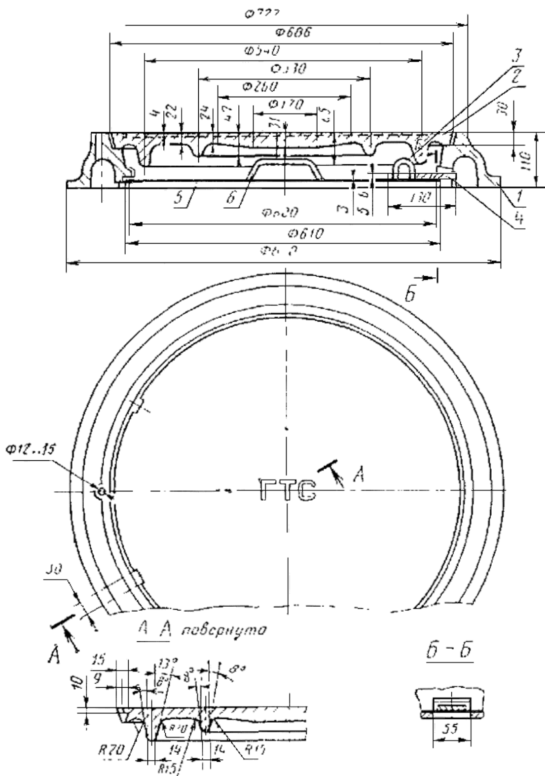
1 - корпус, 2 - верхняя крышка 3 - скоба, 4 - планка запора, 5 - нижняя крышка, 6 - ручка
