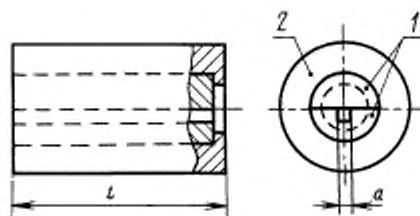
1 — полуматрица; 2 — обойма
