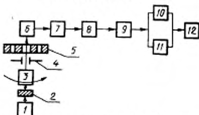
Блок-схема установки
